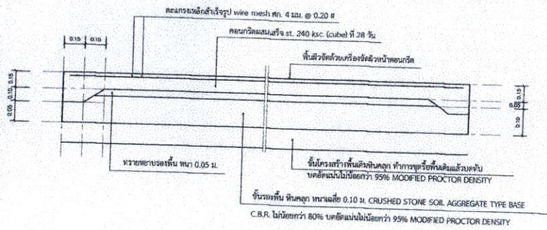
รูปตัดตามยาว พื้นสนาม GS
