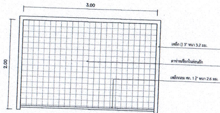
แบบประตูฟุตบอล
