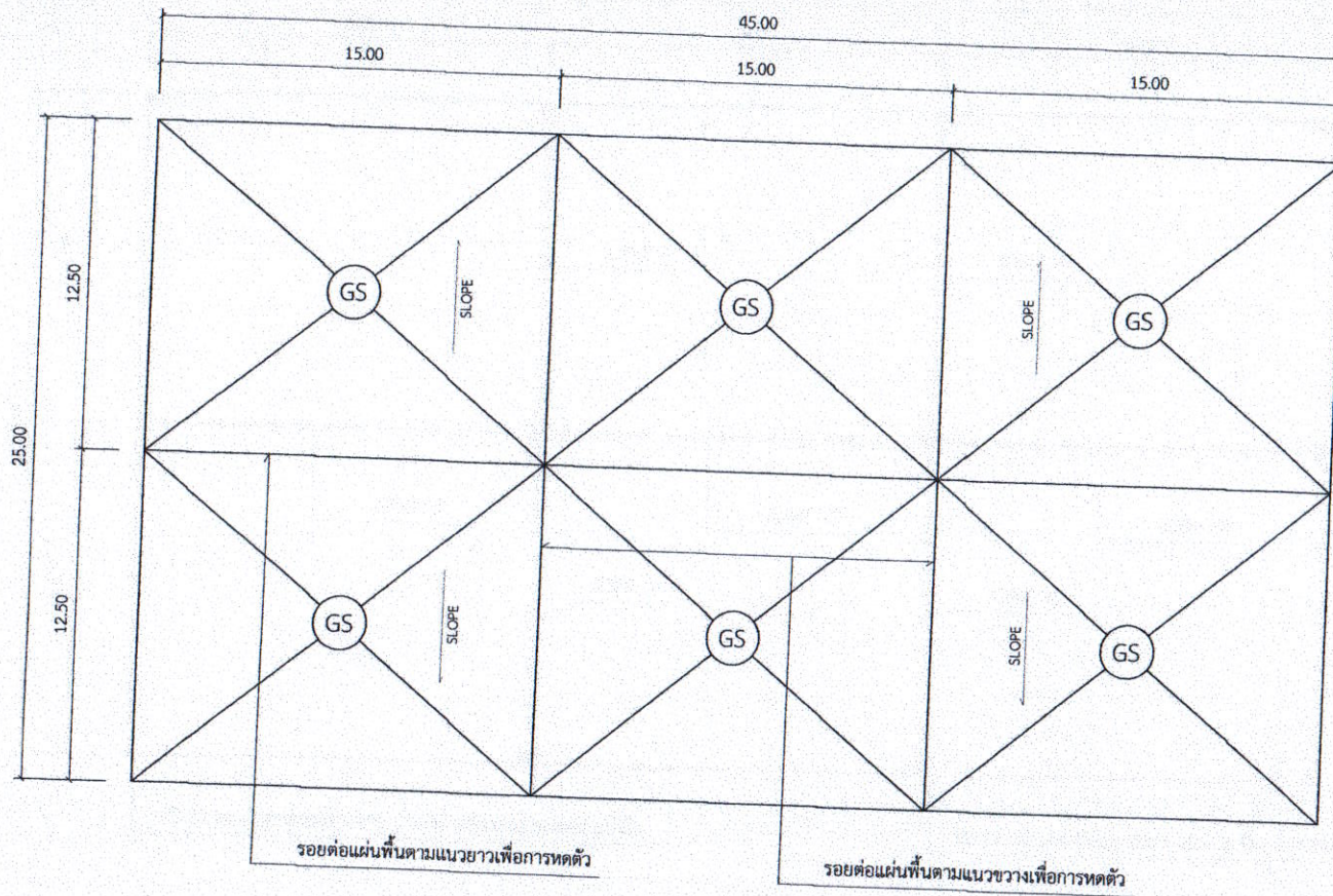
แปลนโครงสร้างพื้นสนามฟุตบอล มาตราส่วน 1 : 200
