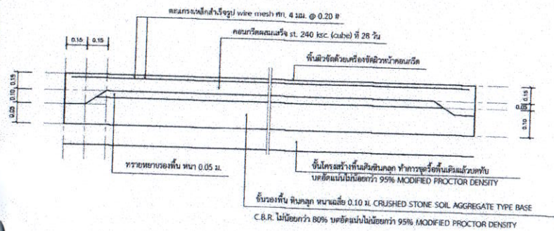
รูปตัดตามขวาง พื้นสนาม GS
